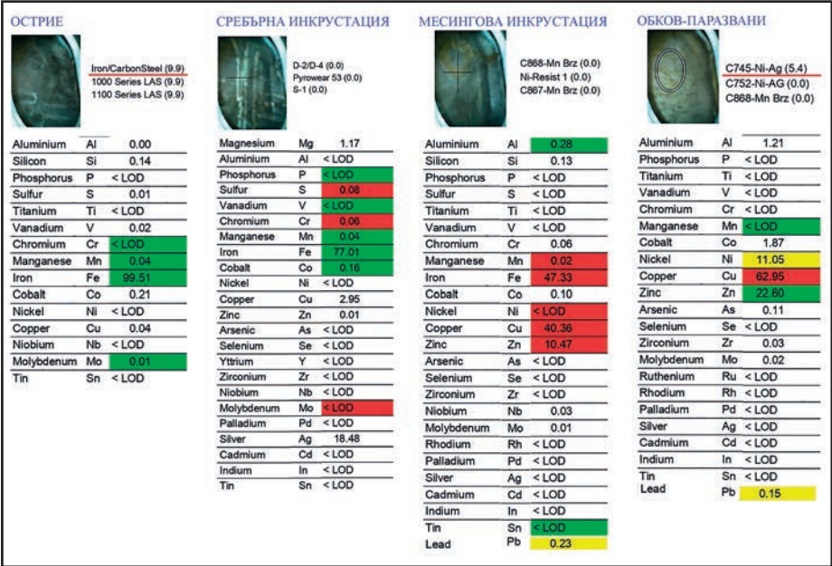
Фиг. 3. Ятаган на Иван Кулин – данни от спектрален анализ / личен архив
