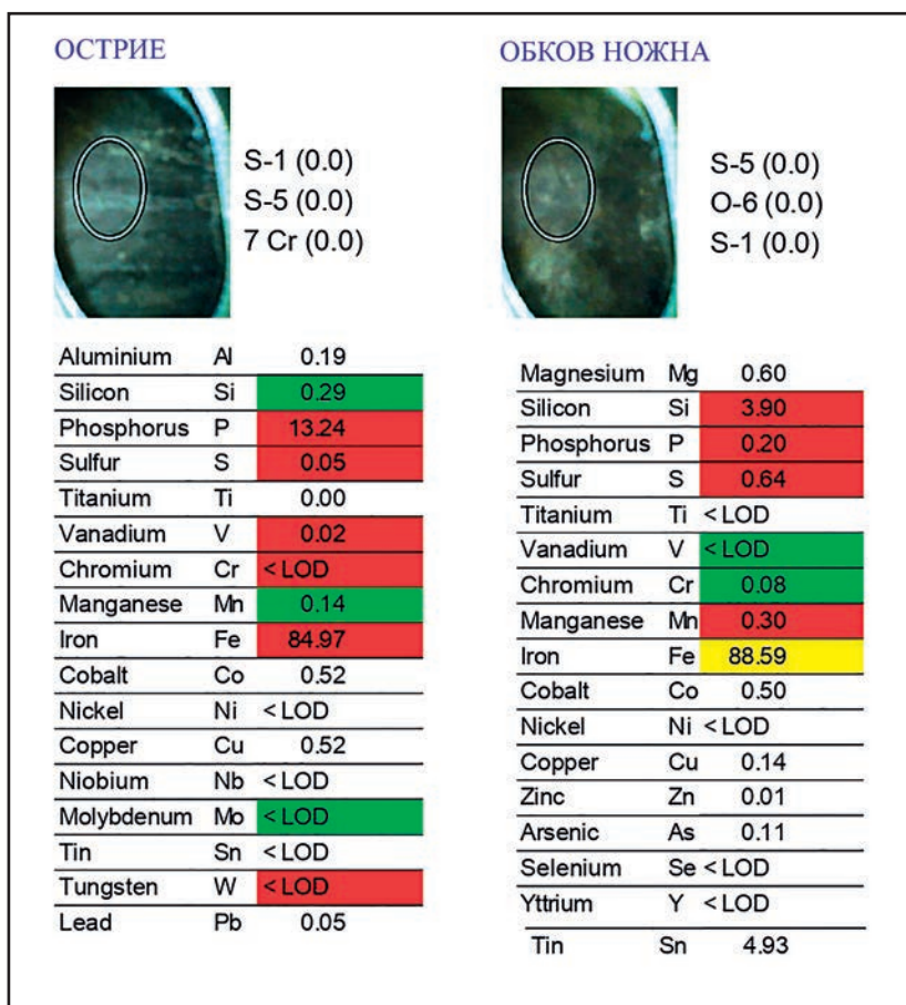
Фиг. 6. Нож-ятаган на Стоян Заимов – данни от спектрален анализ / личен архив
