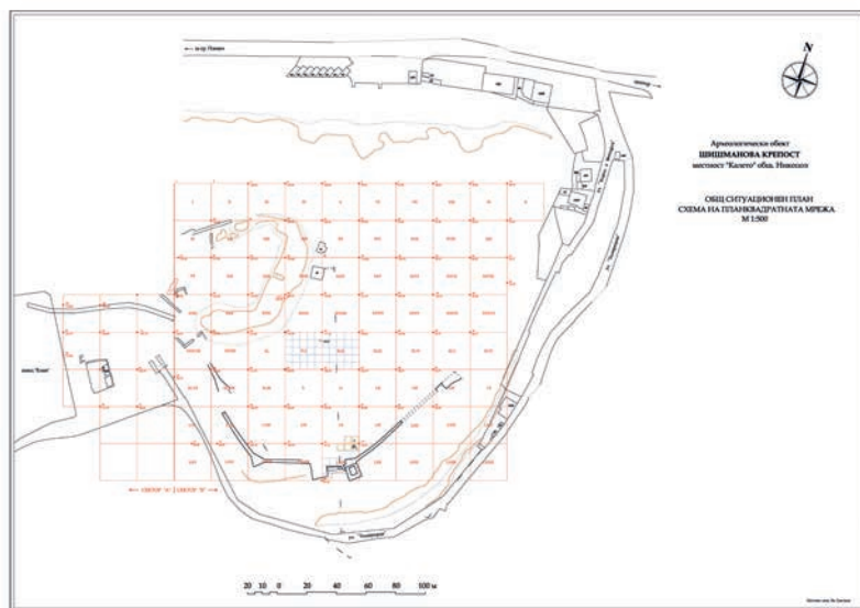
Обр. 2. Общ ситуационен план на Никополска крепост от археологическите проучвания
